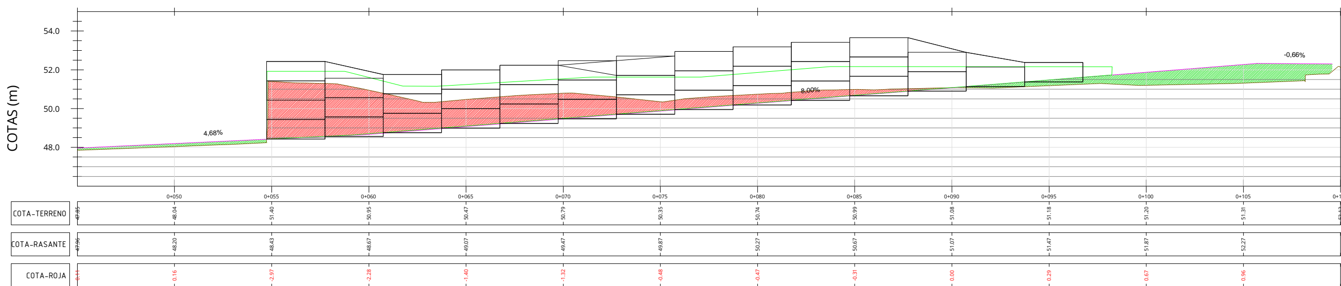
Perf. Longitudinal - Sendero eje
